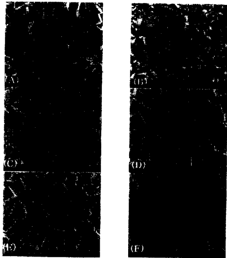
그림 2. 메탄농도에 따른 다이아몬드 박막의 표면 형상
