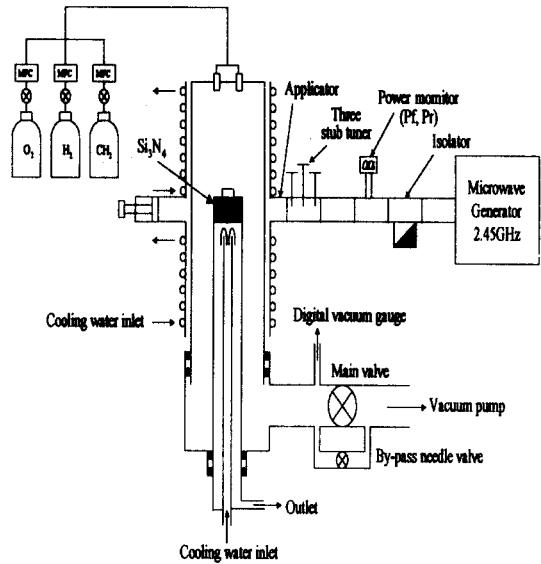
그림 1. 실험장치의 개략도
