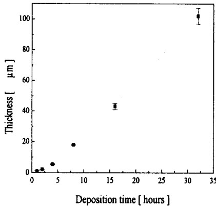
그림 8. 증착시간에 따른 두께변화
