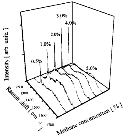
그림 3. 메탄농도에 따른 Raman spectra
