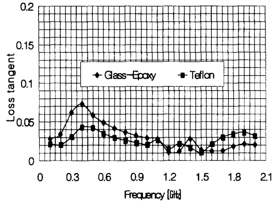
그림 6. Glass-Epoxy와 Teflon 기판의 Loss tangent
