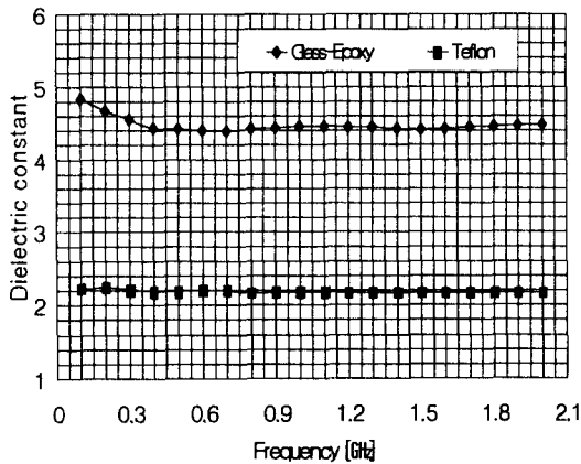
그림 5. 주파수 변화에 따른 Glass-Epoxy와 Teflon 기판의 유전상수
