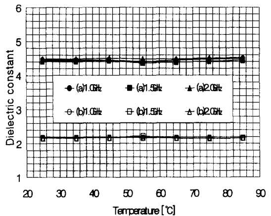
그림 7. 온도 변화에 따른 기판의 유전상수 : (a) Glass-Epoxy (b) Teflon
