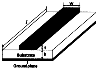
그림 1. 마이크로스트립 라인의 구조 Fig. 1. Structure of microstrip line
