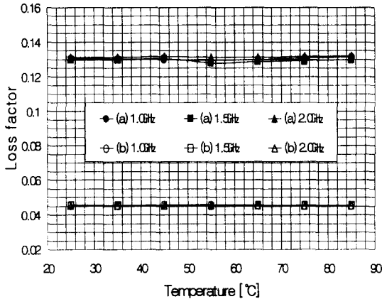
그림 8. 온도 변화에 따른 기판의 손실계수 : (a) Glass-Epoxy (b) Teflon
