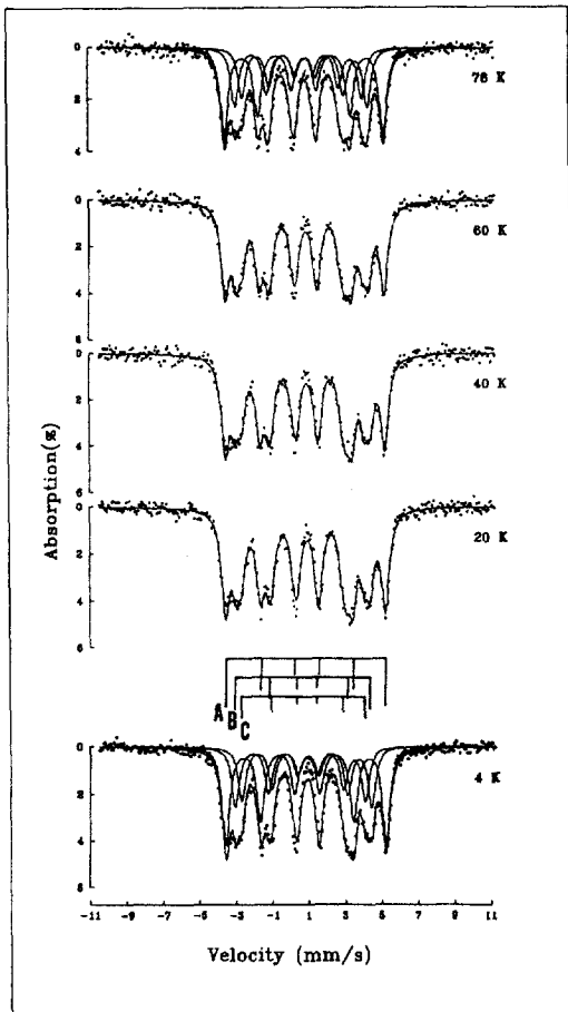
그림 2. 4K에서 78K사이의 다양한 온도에서 Fe_7Se_8 에 대해 취한 뫼스바우어 스펙트럼.
