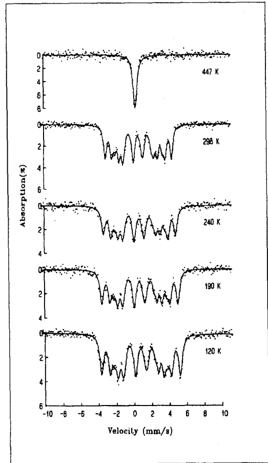
그림 3. 120K에서 447K사이의 다양한 온도에서 Fe_7Se_8 에 대해 취한 뫼스바우어 스펙트럼.
