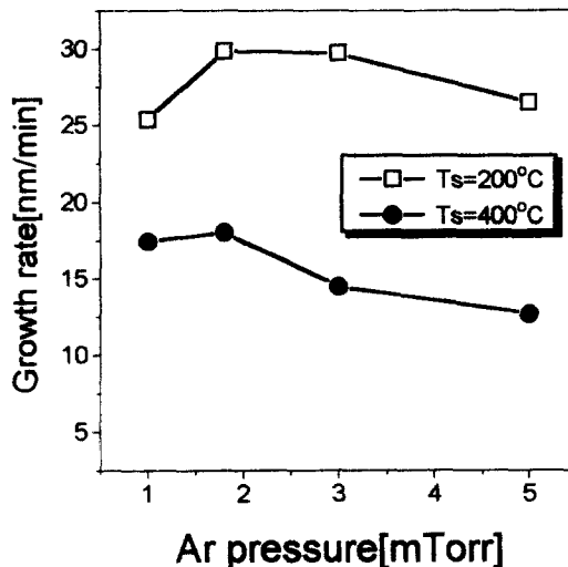
그림 2. Ar 가스압에 따른 성장속도 변화
