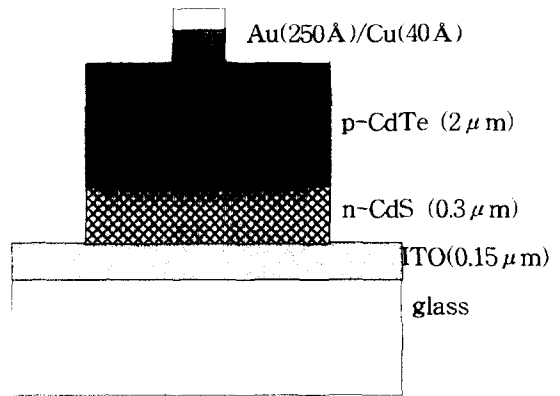
그림 1. CdTe/CdS 태양전지 구조 Fig 1. Structure of CdTe/CdS solar cell
