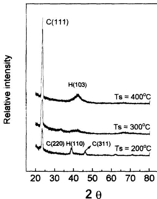
그림 3. 기판온도에 따른 X-선 회절분석
