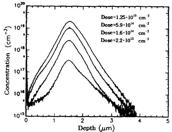
그림 9. 에너지 1.5 MeV 에서 서로 다른 dose로 인 이 주입된 SIMS-profile. Fig. 9. SIMS-profiles of implanted phosphorus ions with different dose at 1.5 MeV.
