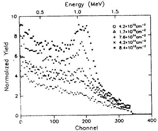
그림 4. 에너지 2 MeV에서 서로 다른 dose로 이온 주입후의 channelingspectra.
