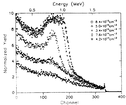
그림 5. 에너지 3 MeV에서 서로 다른 dose로 이온 주입후의 channelingspectra.
