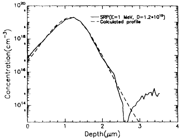
그림 11. 계산된 4개의 moments로 부터 재구성한 profile과 SRP의 비교.
