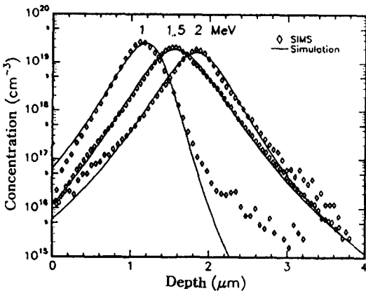
그림 10. 이온 주입된 phosphorus 이온의 측정된 SIMS-data와 simulation-profile의 비교.
