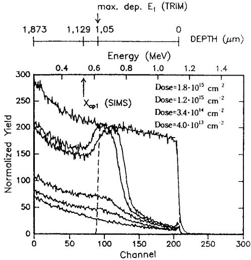
그림 2. 에너지 1 MeV에서 서로 다른 dose로 이온 주입후의 channelingspectra.
