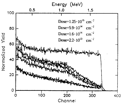
그림 3. 에너지 1.5 MeV에서 서로 다른 dose로 이온 주입후의 channelingspectra.
