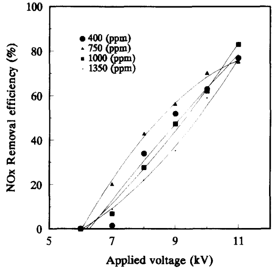
그림 7. 초기농도에 따른 NO x 제거 효율 Fig. 7. Dependence of NO x Removal efficiency on initial concentration
