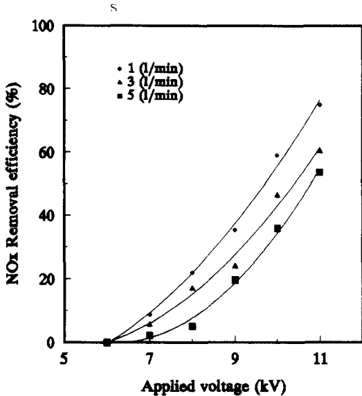
그림 6. 가스유량에 따른 NO x 제거 효율 Fig. 6. Dependence of NO x Removal efficiency on gas flow rate
