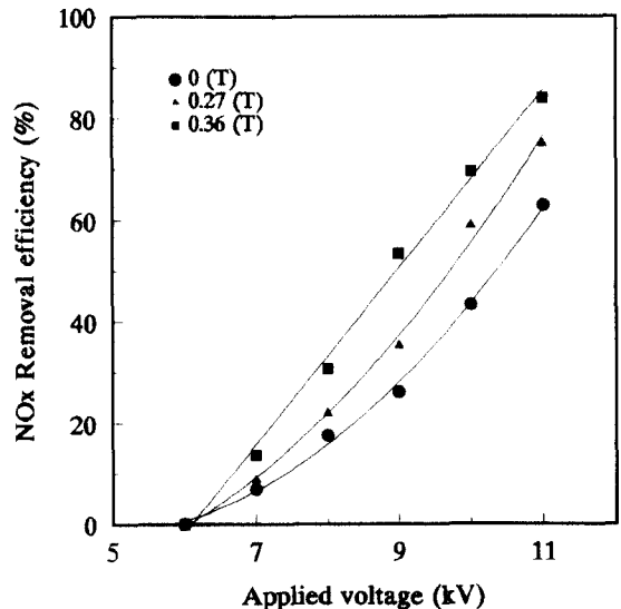
그림 8. 자속밀도에 따른 NO x 의 제거 효율 Fig. 8 Dependence of NO x Removal efficiency on magnetic flux density
