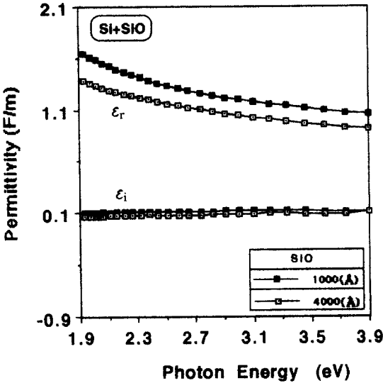
그림 8. 광자에너지에 따른 SiO (A 1 ,A 1 ) 필름의 유전율 ε r , ε i
