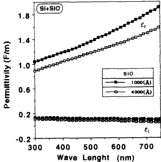
그림 6. 파장에 따른 SiO(A 1 , A 4 ) 필름의 유전율 \epsilon_r, \epsilon_i
