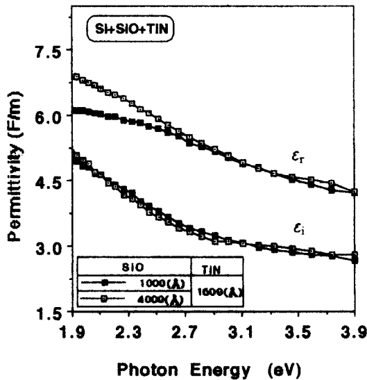
그림 9. 광자 에너지에 따른 SiO/TiN (B 1 ,B 4 ) 필름의 유전상수 ε r , ε i
