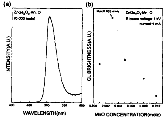
그림 3. 진공 분위기에서 소성된 ZnGa 2 O 4 :Mn 2 O 형광체의 (a) CL 스펙트럼과 (b) MnO의 몰비에 따른 CL 휘도
