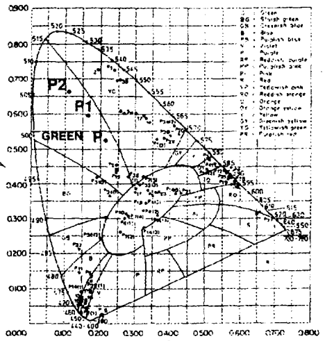
그림 4. 진공과 Ar 분위기에서 소성된 ZnGa 2 O 4 :Mn 2 O의 색좌표
