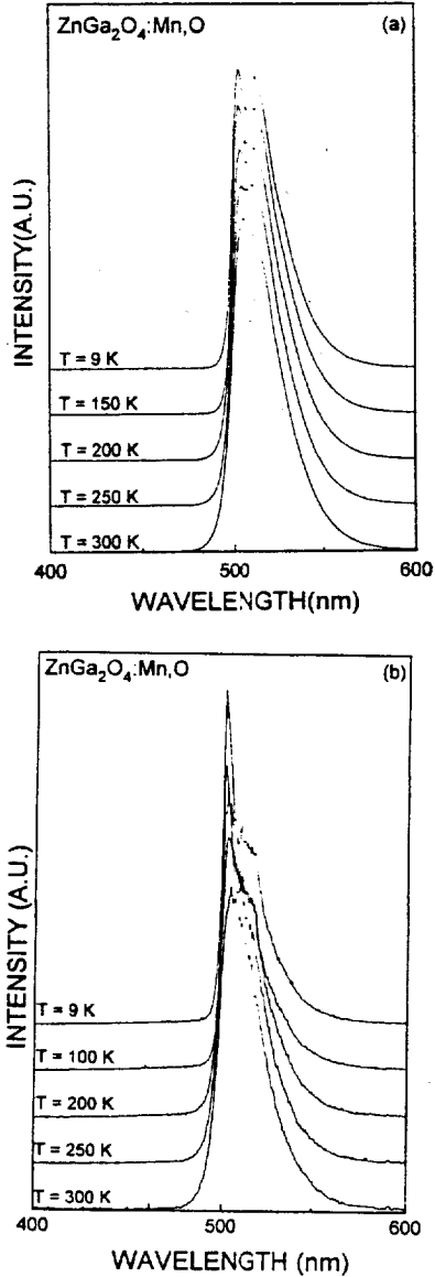
그림 5. 진공 (a)과 Ar (b) 분위기에서 제작된 ZnGa_2O_4:Mn,O 의 온도 변화에 따른 PL 스펙트럼
