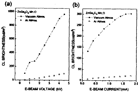
그림 2. Ar과 진공 분위기에서 소성된 ZnGa 2 O 4 :Mn 2 O의 전압 (a)과 전류 (b)에 따른 CL 휘도
