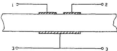
그림 11. 단일 이중 결합 필터의 구조 Fig. 11. Configuration of a double-coupled filter.
