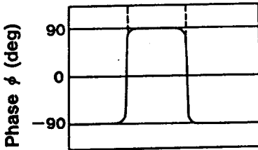
그림 4. 세라믹스 공진자의 주파수 특성 Fig. 4. Frequency characteristics of a ceramic resonator.
