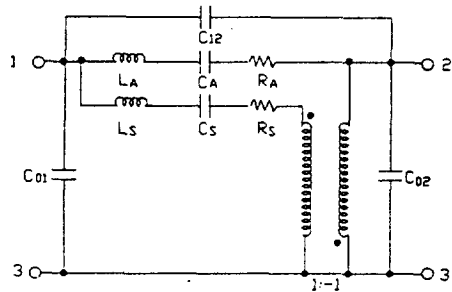
그림 13. 단일 이중 결합 필터의 전기 동가회로 Fig. 13. An electrical equivalent circuit of a double-coupled filter.
