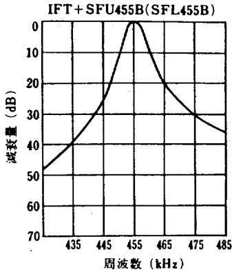
그림 7. 링-도트 분할 전극형 필터의 주파수 특성
