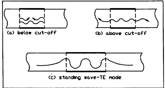
그림 2. 에너지 포획 현상 Fig. 2. Energy-trapped phenomenon.
