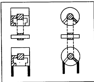
그림 1. 에너지 포획형 공진자의 구조 Fig. 1. Configuration of energy-trapped resonators
