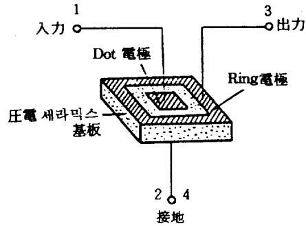
그림 5. 링-돛트 분할 전극형 필터의 구조 Fig. 5. Configuration of a ring-dot split electrode type filter.
