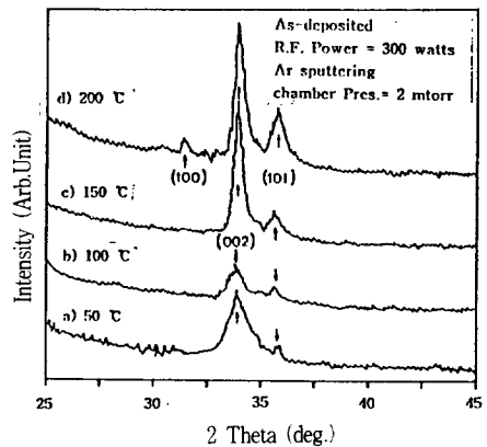
그림 4. 기판온도에 따른 ZnO 박막의 XRD spectra (as-deposited, 고주파전력 = 300 watts, Ar 스퍼터링, 챔버압력 = 2 mtorr)
