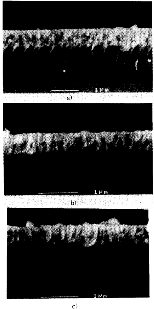
그림 7. ZnO 박막의 단면 SEM 사진
