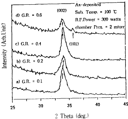
그림 5. 가스 유량비[(O 2 / (O 2 + Ar)) = G.R.]의 증가에 따른 ZnO 박막의 XRD spectra ( as-deposited, 기판온도 = 100 ℃, 고주파 전력 = 300 watts, 챔버압력 = 2 mtorr )
