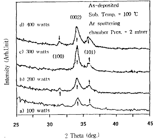
그림 6. 인가 고주파 전력에 따른 ZnO 박막의 XRD spectra( as-deposited, 기판온도 = 100 ℃, Ar 스퍼터링, 챔버압력 = 2 mtorr )
