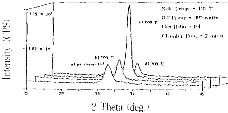
그림 8. 열처리 전후 ZnO 박막의 XRD spectra( 기판온도 = 150 ℃, 고주파 전력 = 300 watts, Gas Ratio = 0.4, 챔버압력 = 2 mtorr ) a) as-deposited, b) 500 ℃, c) 600 ℃, d) 700 ℃
