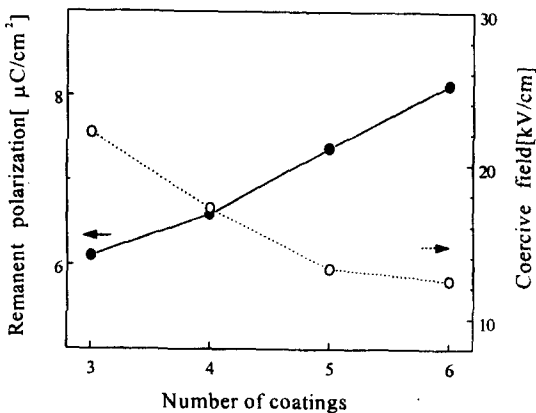
그림 9. PZT 이중층 박막의 코팅횟수에 따른 잔류 분극 및 항전계 Fig. 9. Remanent polarization and coercive field of PZT heterolayered thin films as a function of the number of coatings
