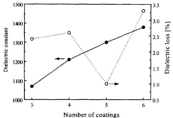
그림 7. PZT 이중층 박막의 코팅횟수에 따른 유전 상수 및 유전손실 [1kHz] Fig. 7. Dielectric constant and dielectric loss of PZT heterolayered thin films as a function of the number of coatings [1kHz]
