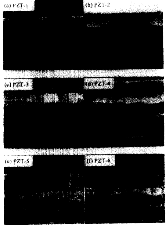
그림 4. PZT 이종층 박막의 단면 SEM 사진
