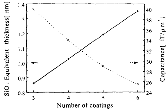
그림 10. PZT 이중층 박막의 \text{SiO}_2 환산두께 및 정전용량 Fig. 10. \text{SiO}_2 equivalent thickness and capacitance of PZT heterolayered thin films
