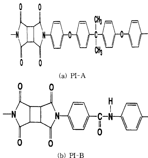
그림 1. 사용한 2 종류의 고분자의 분자구조.
