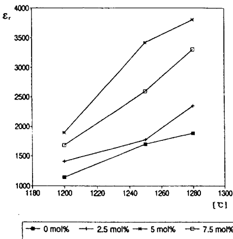
그림 3. 소결온도 및 Ba 첨가량에 따른 유전상수 Fig. 3. Dielectric constant with Ba additions and sintering temp.
