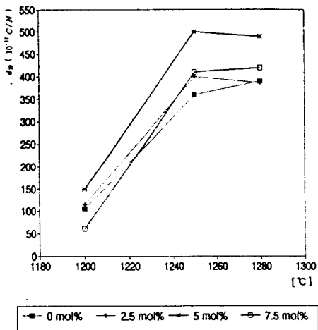
그림 6. 소결온도 및 Ba 첨가량에 따른 압전계수 Fig. 6. Piezoelectric coefficient with Ba addition and sintering temp.
