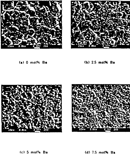
사진 1. Ba 첨가량에 따른 미세구조 Photo. 1. Microstructure with Ba additions.
