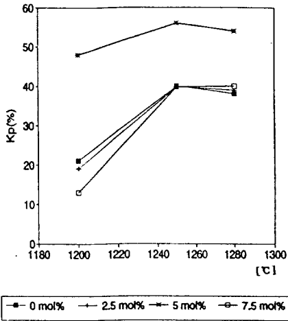
그림 5. 소결온도 및 Ba 첨가량에 따른 전기기계 결합계수
