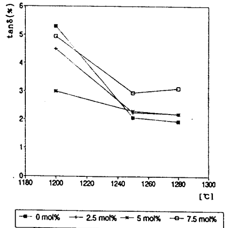
그림 4. 소결온도 및 Ba 첨가량에 따른 유전손 Fig. 4. Dielectric loss with Ba additions and sintering temp.
