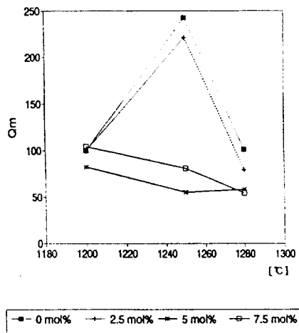
그림 7. 소결온도 및 Ba 첨가량에 따른 기계적 품질계수
