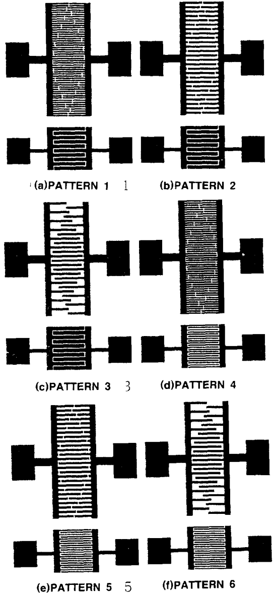
그림 1. SAW 필터의 패턴 Fig. 1. Patterns of SAW filters
