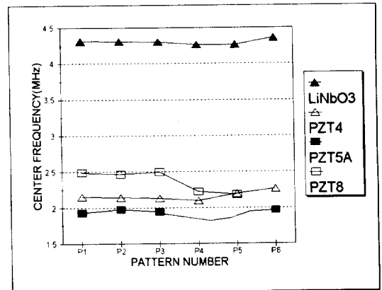
그림 2. 패턴의 중심 주파수 Fig. 2. Center frequency of patterns
