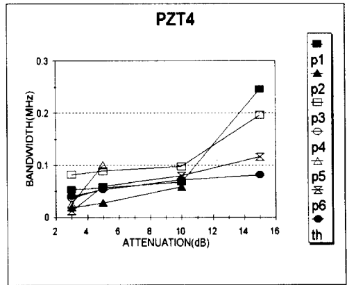
(b) PZT4
