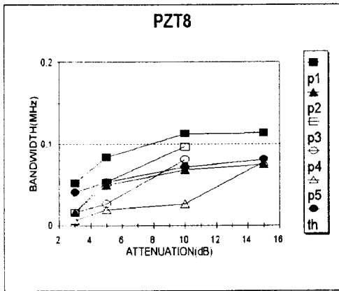
(d) PZT8
