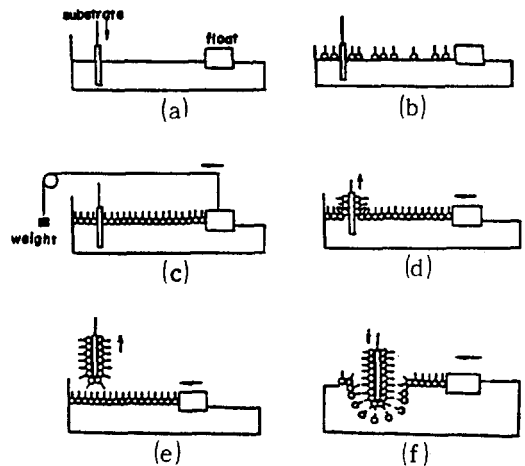
그림 4. Y-type 의 LB막 제작과정 Fig 4. Schematic LB film deposition process of the Y-type.
