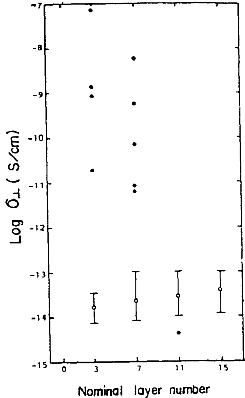
그림 9. LB막의 기판과 수직방향의 도전율 Fig.9. Perpendicular conductivity( \sigma_{\perp} ) vs. nominal layer number of the LB film.
