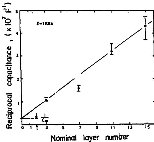
그림 7. LB막의 누적층수와 1/C 과의 관계 Fig.7. Nominal layer number vs. reciprocal capacitance of the LB film.
