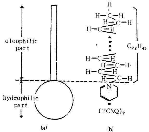
(a) 양친매성 분자 (b) (N-docosyl pyridinium) - TCNQ (1:2) 착체의 분자
