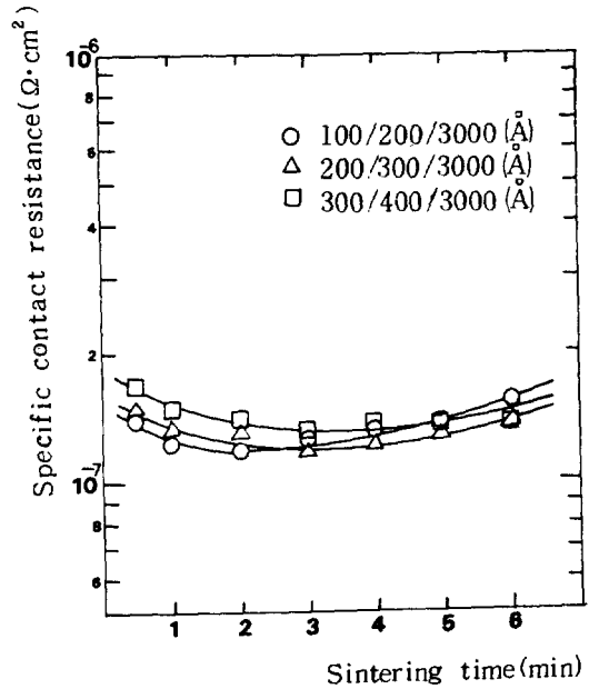
그림 8. 430°C에서 시편 B의 Pd/Ge 두께 변화에 대한 접촉저항
