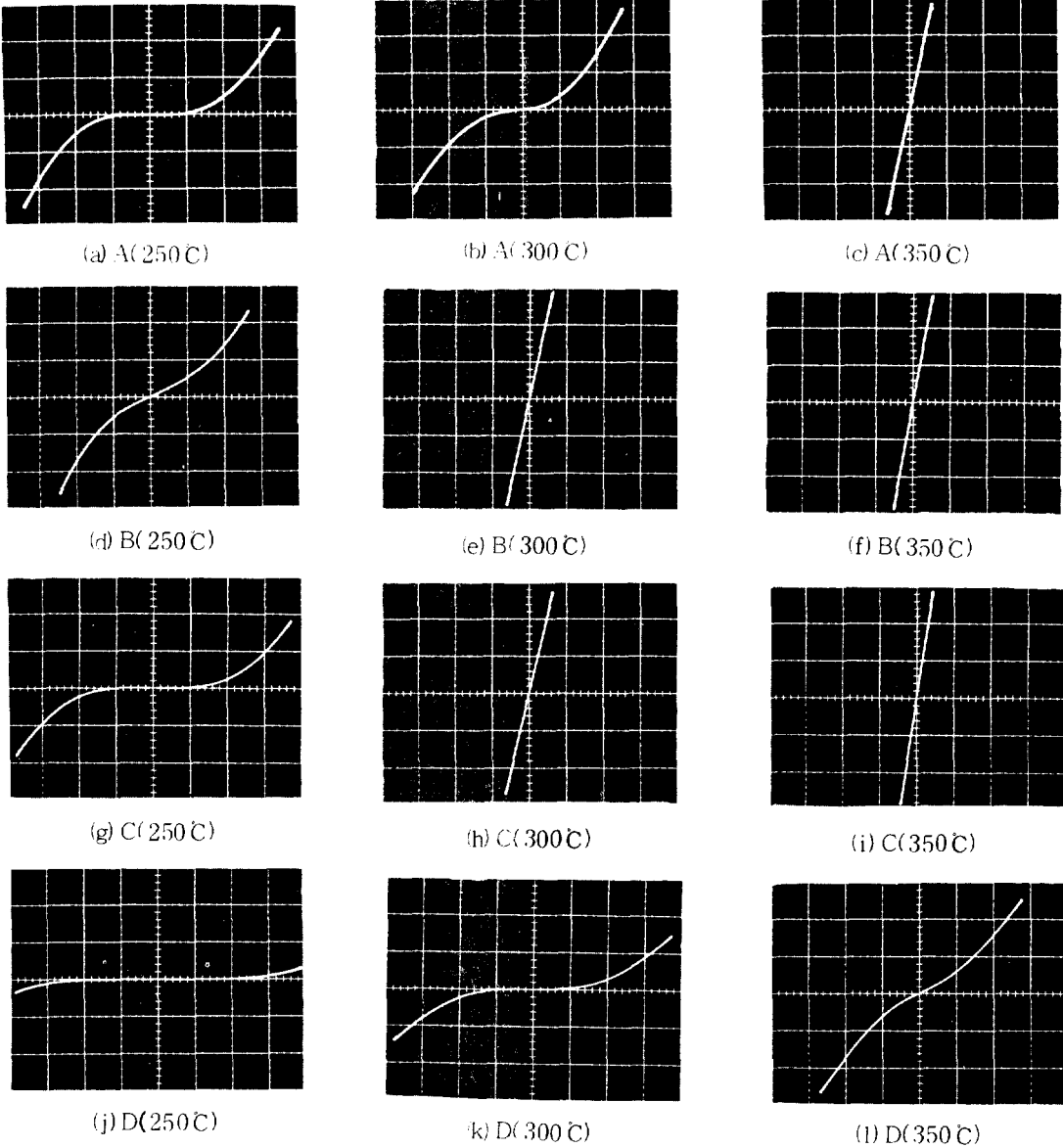
그림 3. 250°C와 350°C 사이에 10분 Sintering 된 시편 A, B, C, D의 ohmic 형성과정에 대한 전류-전압 특성 종축 : 20mA/div. 횡축 : 1V/div.
