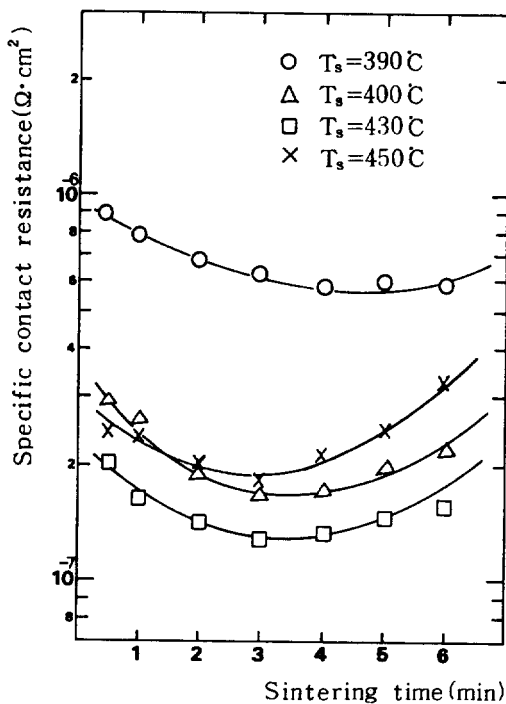
그림 4. 여러가지 sintering 온도에서 sintering 시간에 따른 시편 A의 접촉저항
