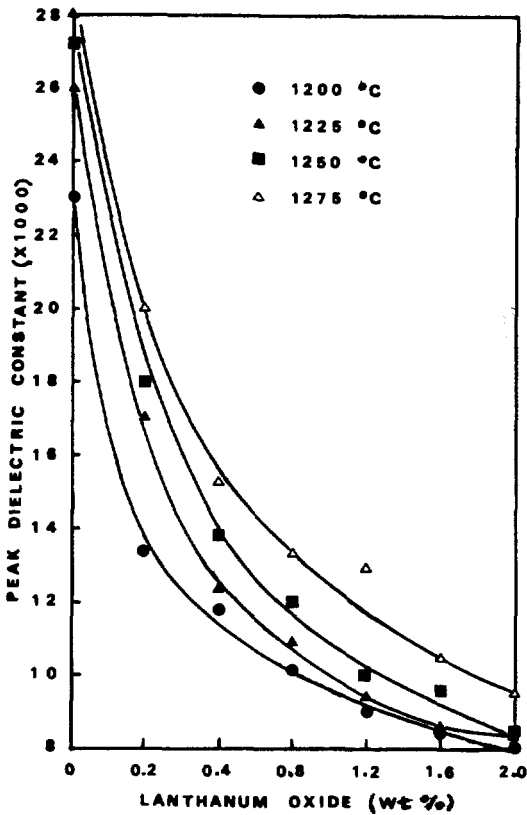
그림 4. La 2 O 3 의 첨가량에 따른 유전상수 최대치의 변화
