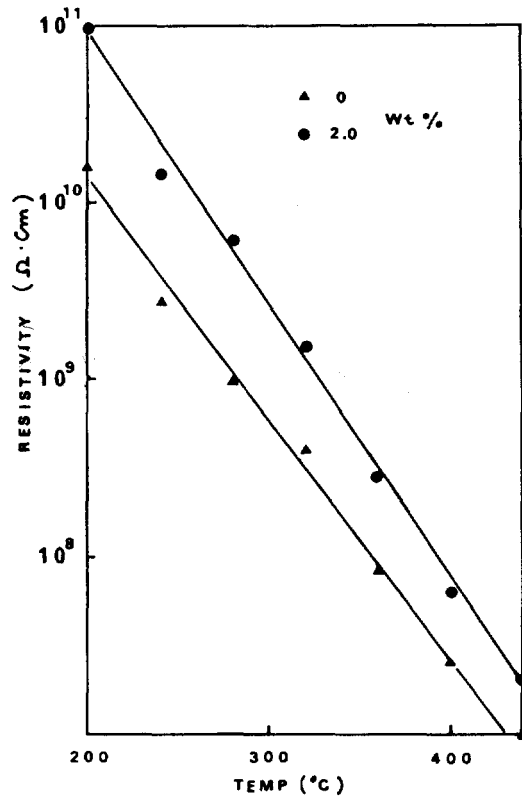
그림 5. La 2 O 3 첨가에 따른 비저항의 변화
