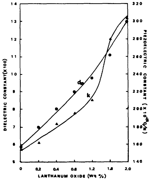
그림 1. La 2 O 3 첨가량에 따른 유전상수와 압전 d 상수
