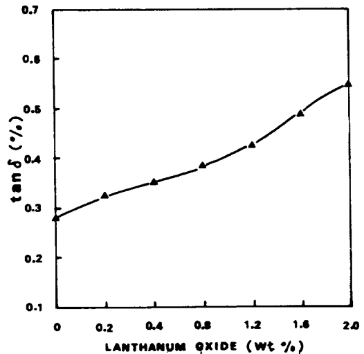
그림 3. La 2 O 3 첨가량에 따른 유전손실의 변화 Fig 3. Variation of dielectric loss(ten δ) with La 2 O 3 addition.
